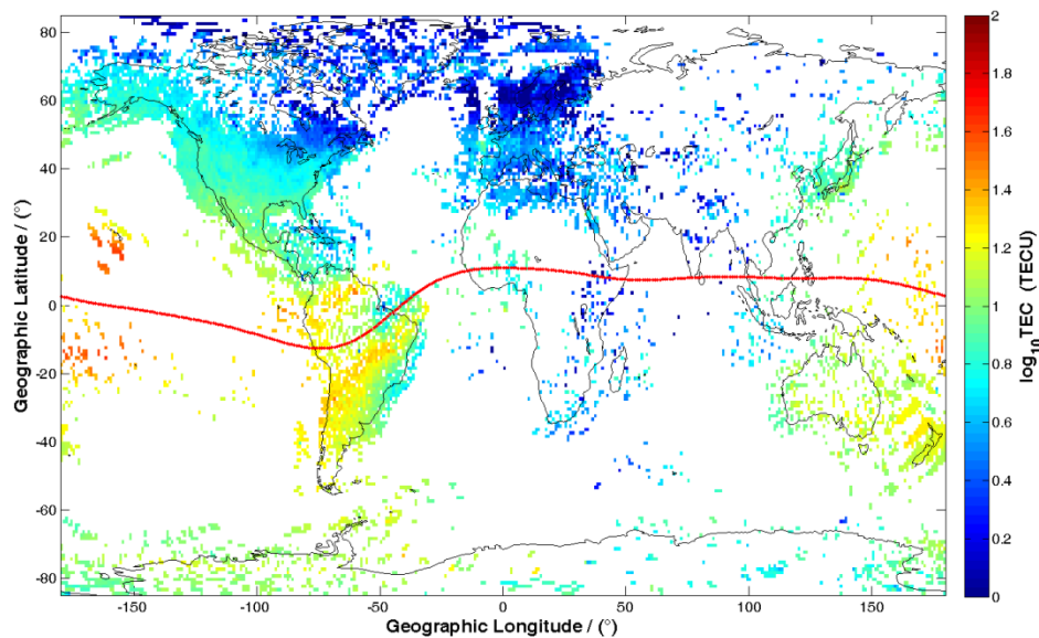
Fig.1 The distribution map of MIT TEC data
