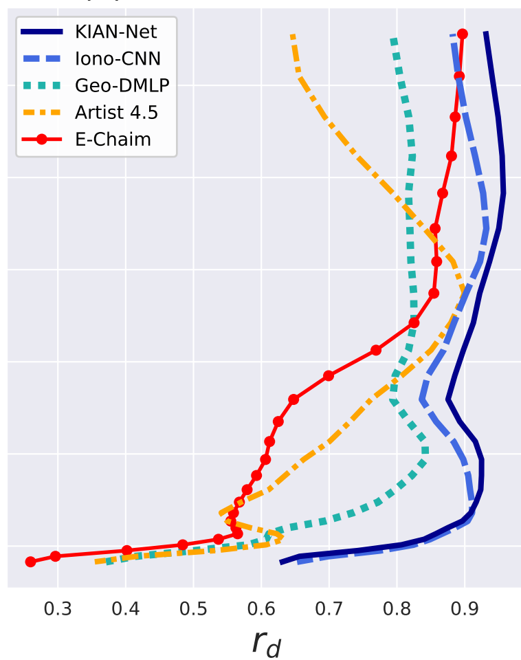
(d) Distance Correlation
