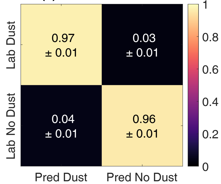
(d) The CNN Classifier
