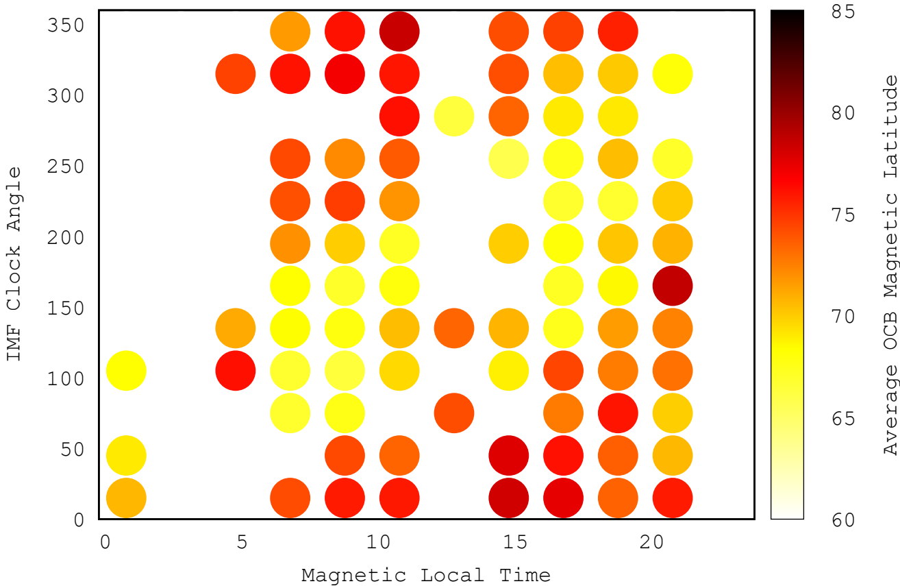
Average OCB latitude versus IMF clock angle (model)
