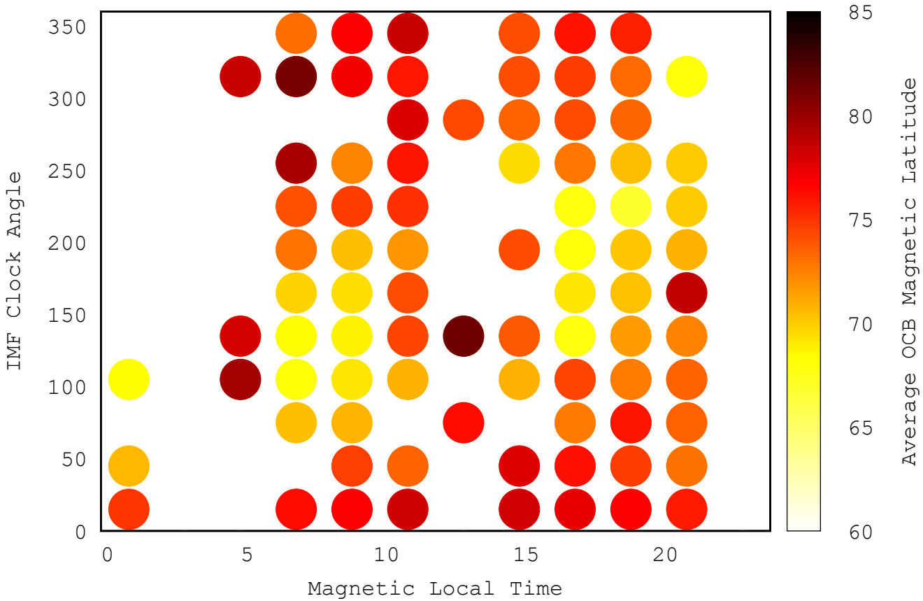
Average OCB latitude versus IMF clock angle (data)
