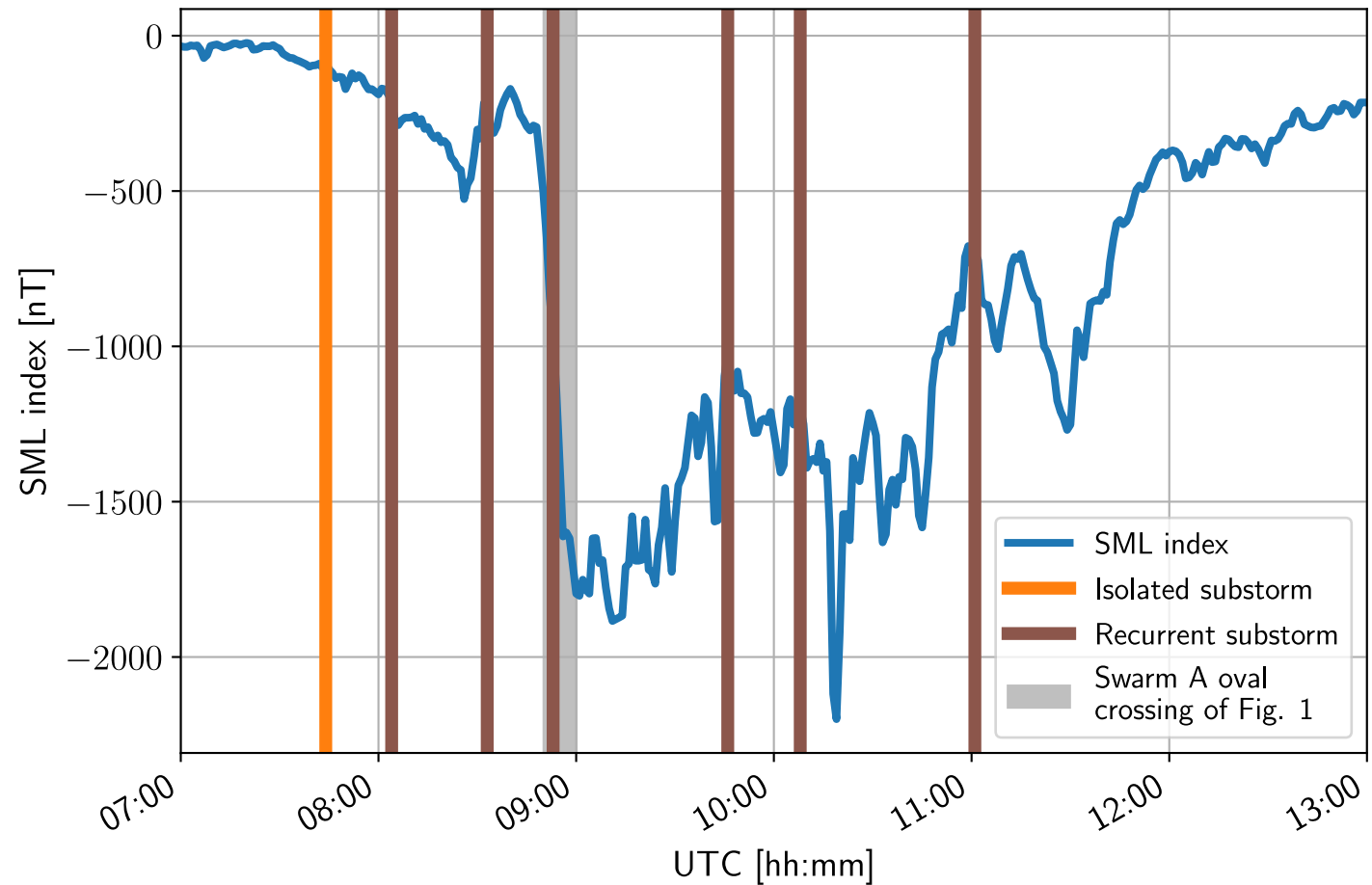
SuperMAG SML index 2015-01-07 07:00–13:00 UT
