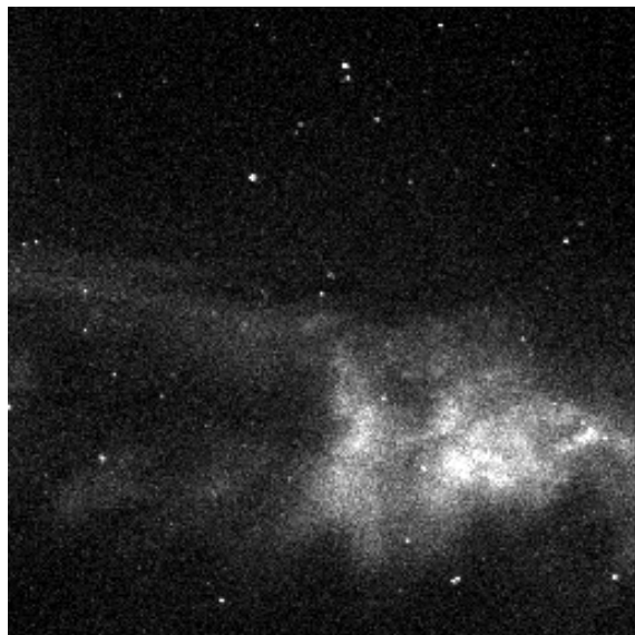
ASK1 N 2 1P 673.0 nm
