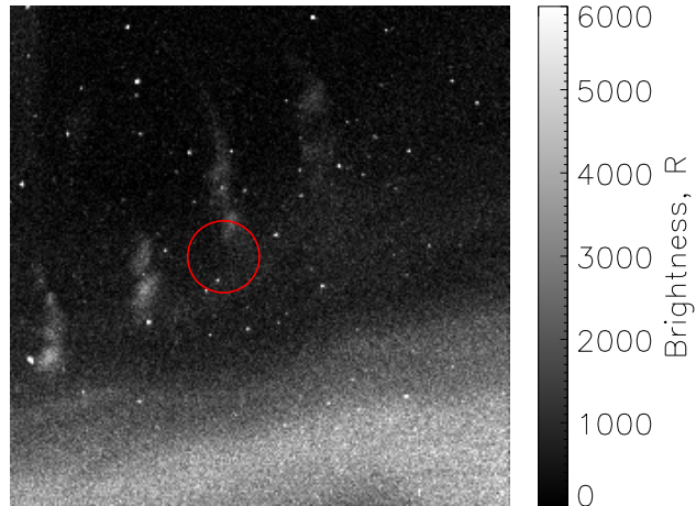
(a) ASK1 N 2 1P 673.0 nm
