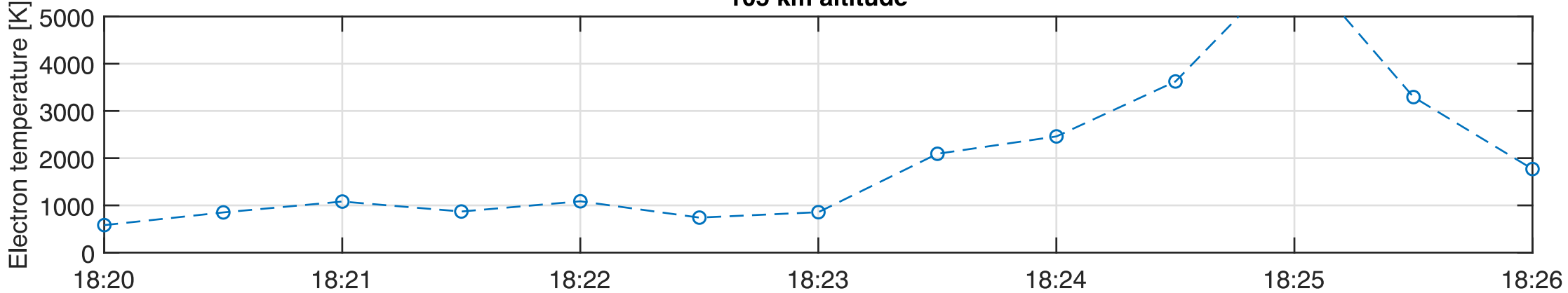
109 km altitude
