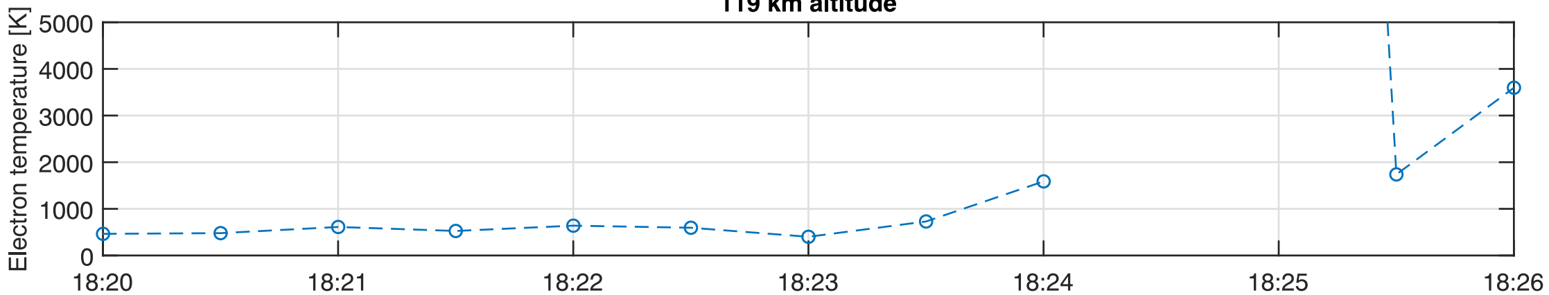
119 km altitude
