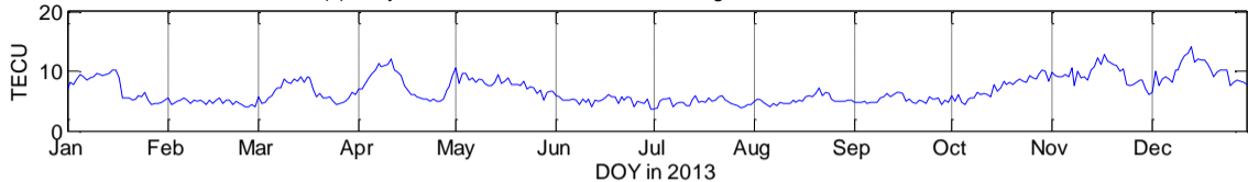
(b) Daily solar F10.7 index
