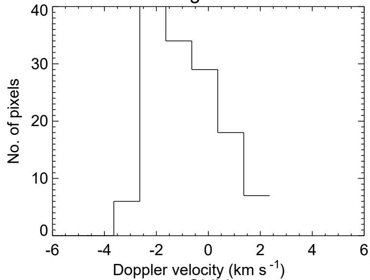
Si IV
