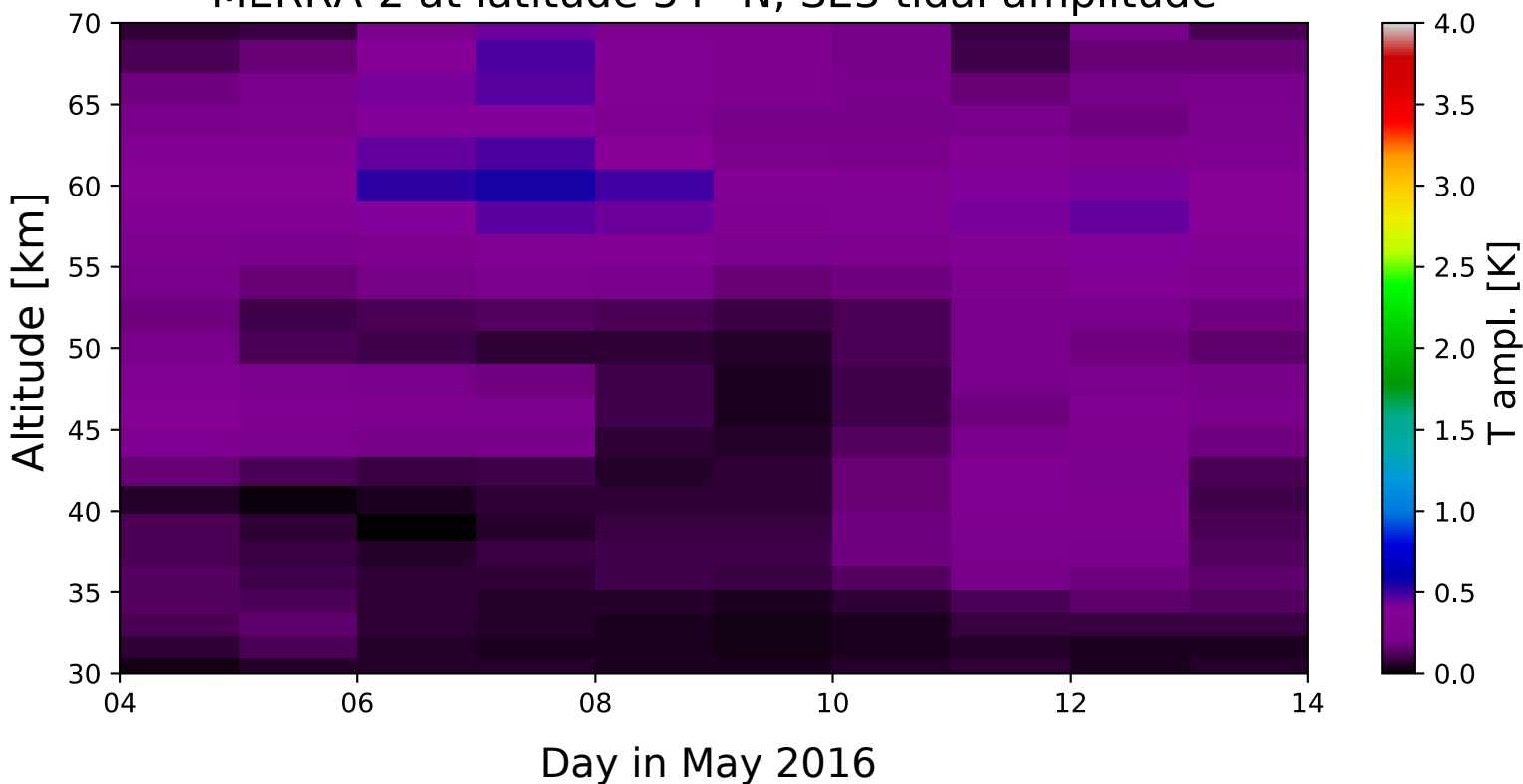
MERRA-2 at latitude 54° N, SE3 tidal amplitude
