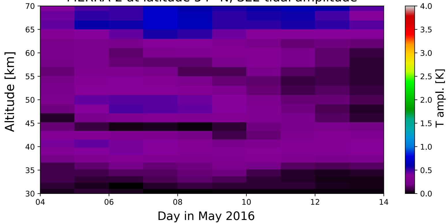
MERRA-2 at latitude 54° N, SE2 tidal amplitude
