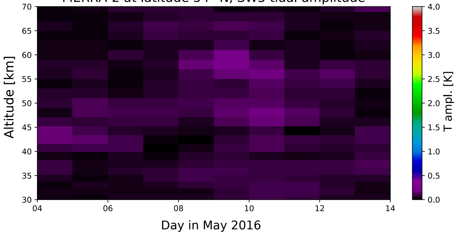
MERRA-2 at latitude 54° N, SW3 tidal amplitude
