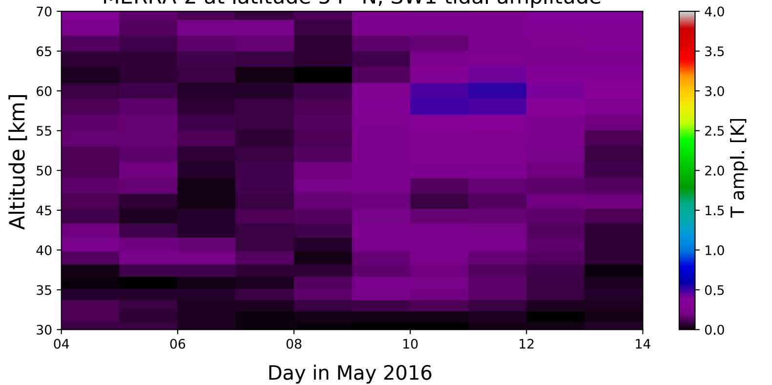
MERRA-2 at latitude 54° N, SW1 tidal amplitude
