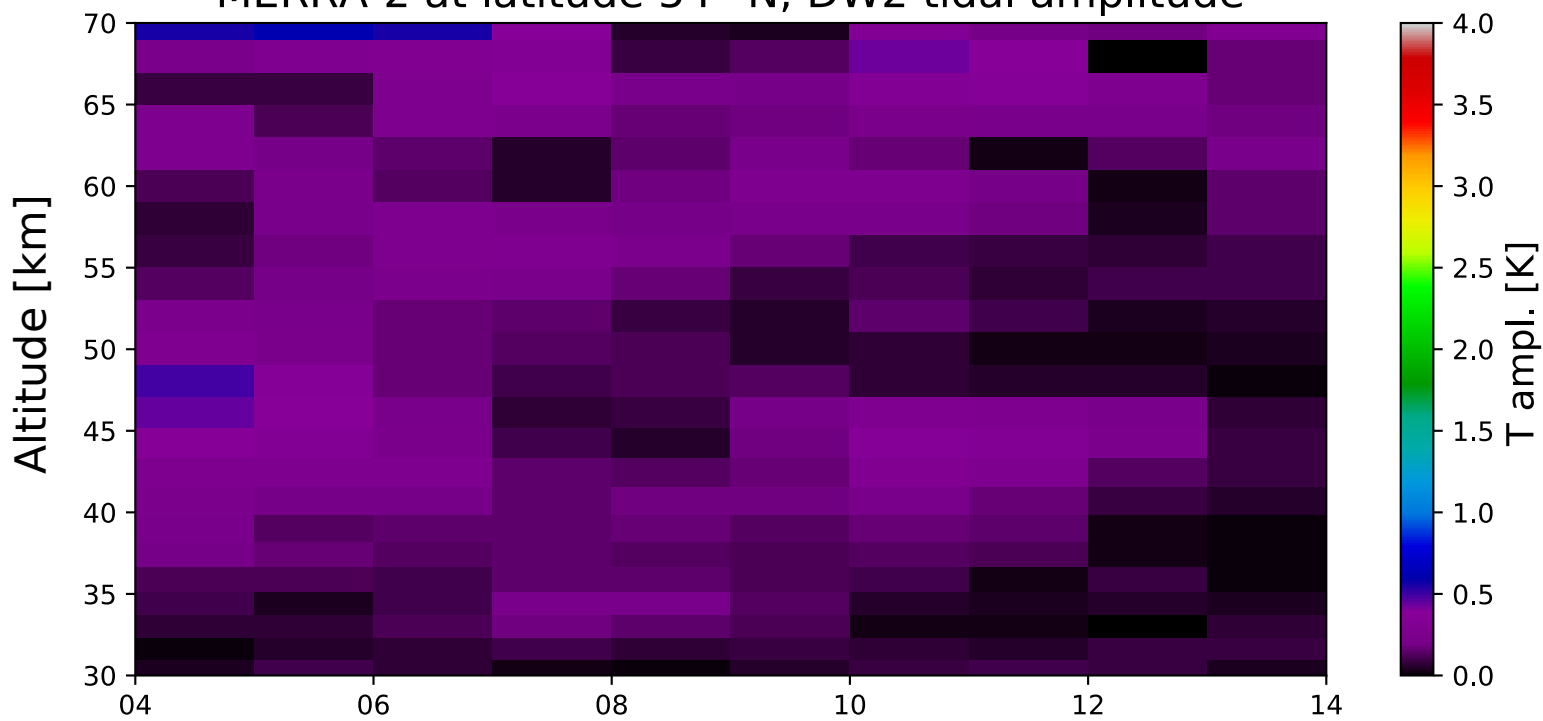
MERRA-2 at latitude 54° N, DW2 tidal amplitude
