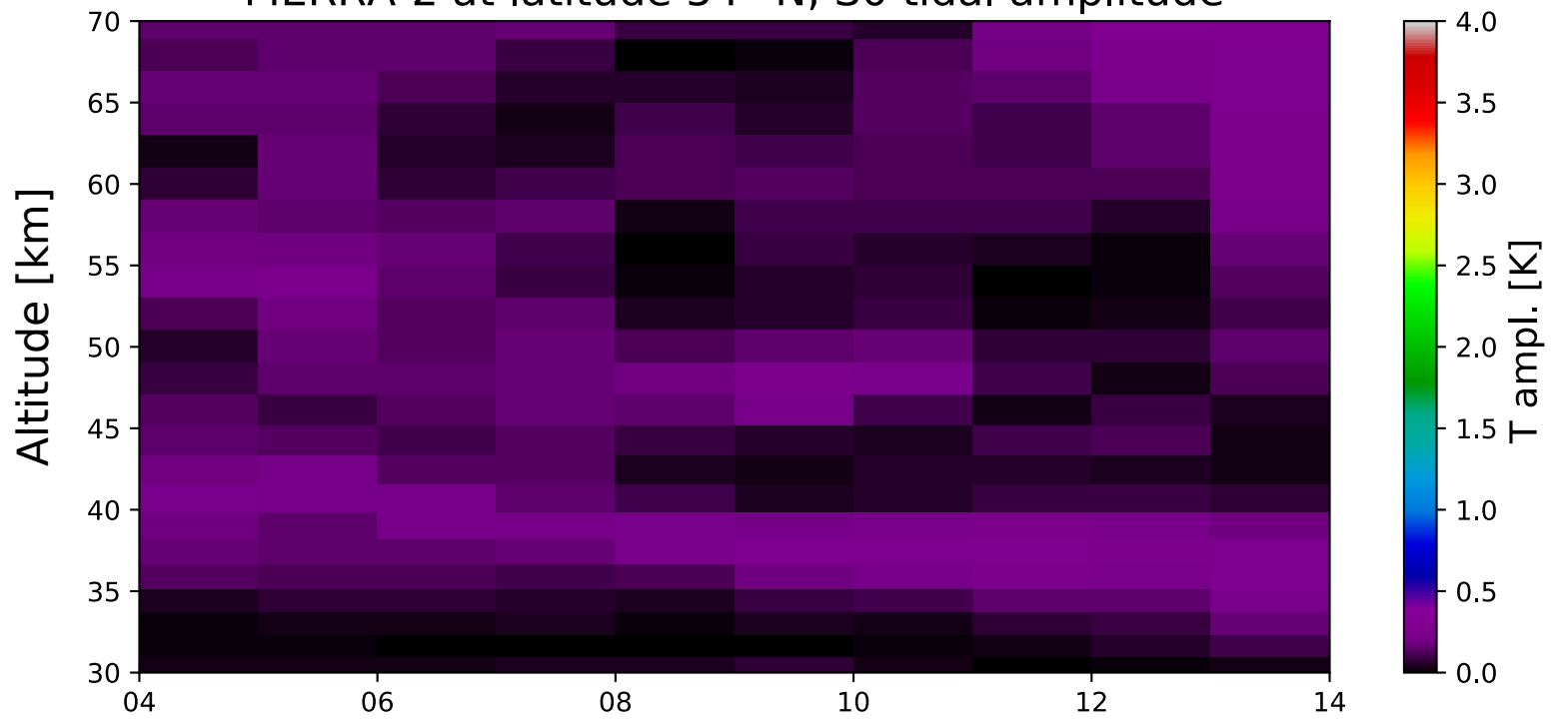
MERRA-2 at latitude 54° N, S0 tidal amplitude
