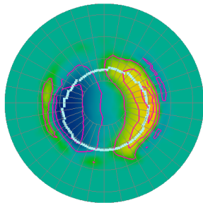
(d) July 16, 03:00 0.25 R_E
