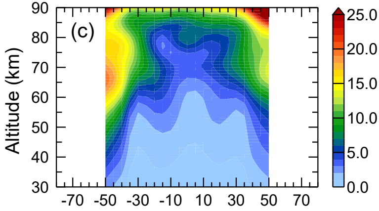
sqrt(Varia of recon_GWSTA) (K 2 )
