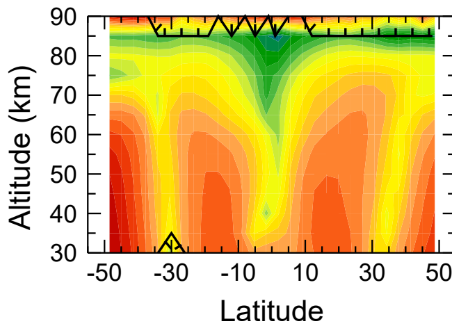
(d) AV: |GWMF| ( \log_{10}\text{Pa} )
