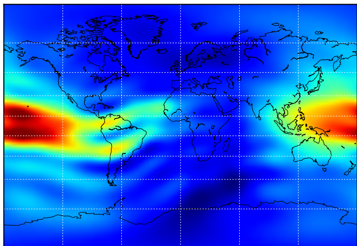
(a) 17/03/2015 02:00 UT
