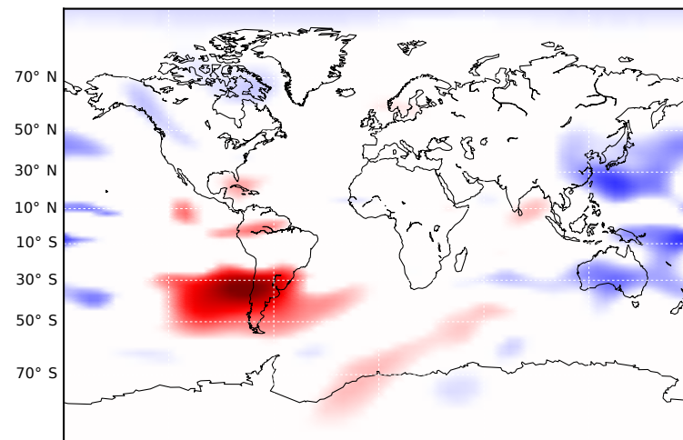
(d) 18/03/2015 02:00 UT
