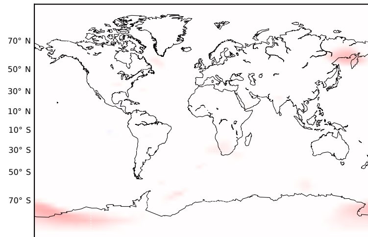
(b) 17/03/2015 02:00 UT
