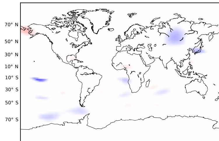
(f) 19/03/2015 02:00 UT
