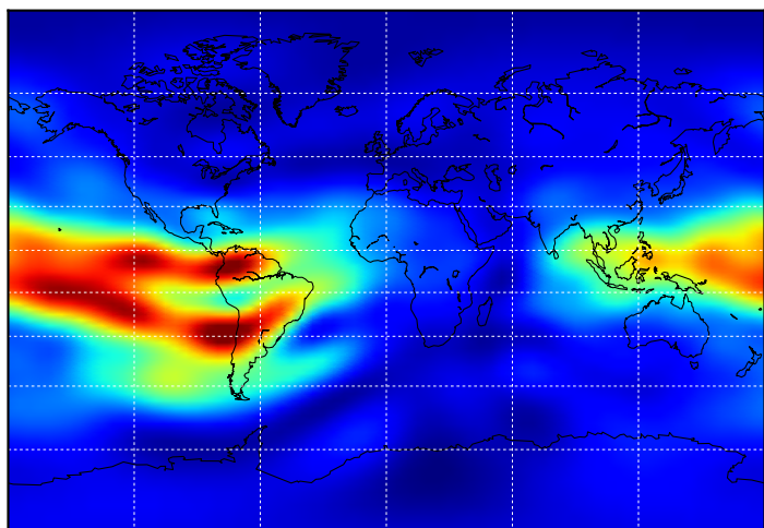
(c) 18/03/2015 02:00 UT
