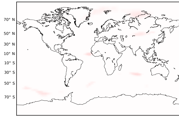
(d) 08/09/2017 02:00 UT
