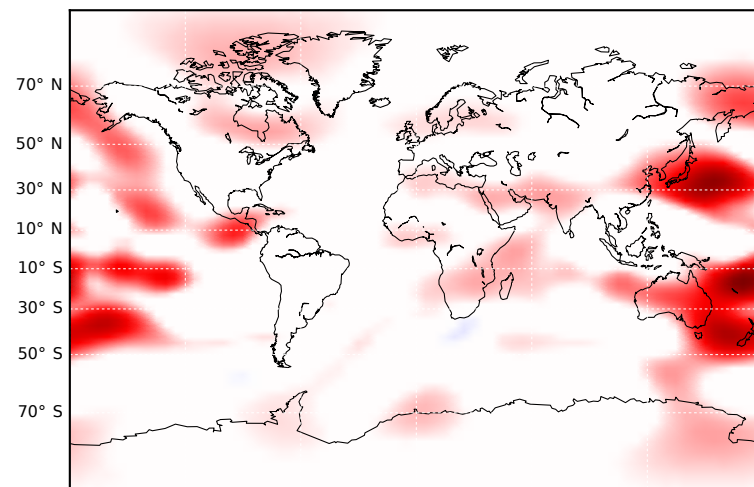
(d) 08/09/2017 02:00 UT
