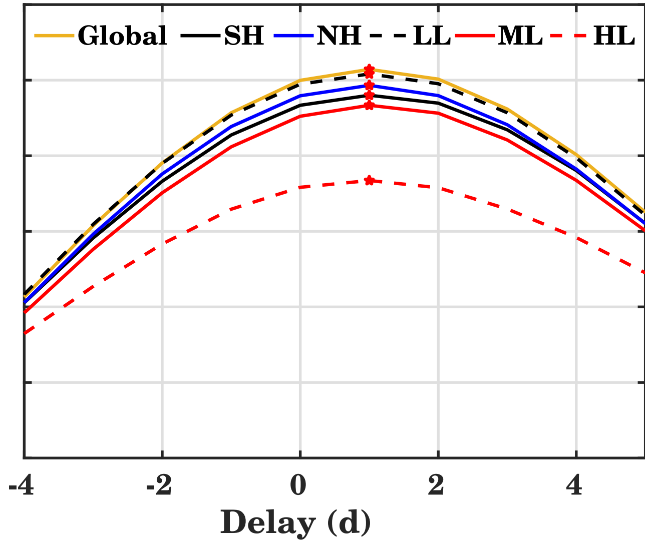
(b) TEC-Mg II index
